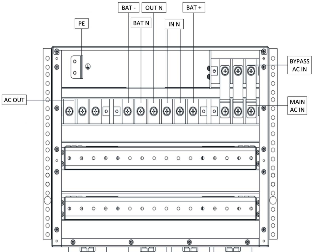
Coway PowerUnit M e40/e50, схема подключения
