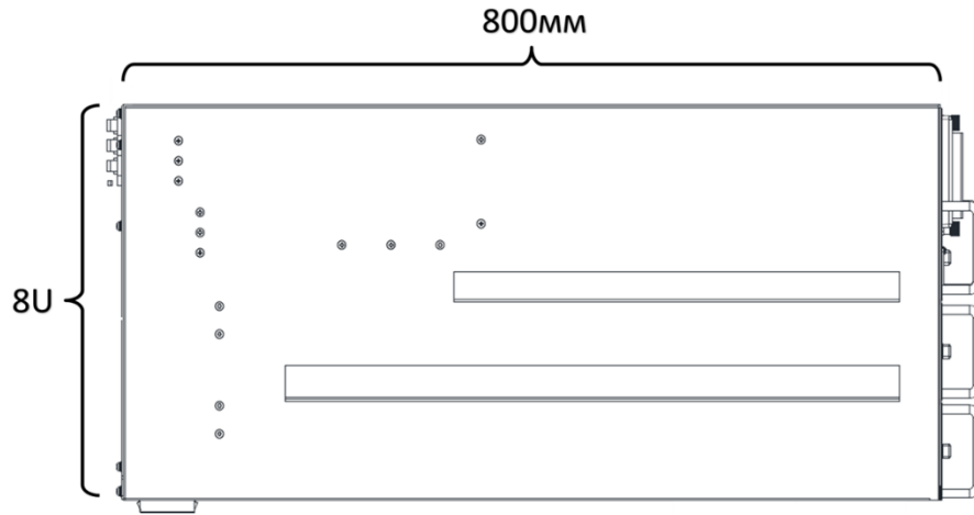
Coway PowerUnit M e40/e50, вид сбоку
