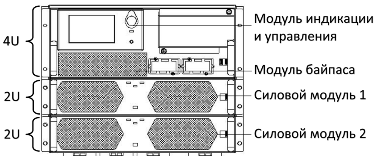
Coway PowerUnit M e40/e50, вид спереди
